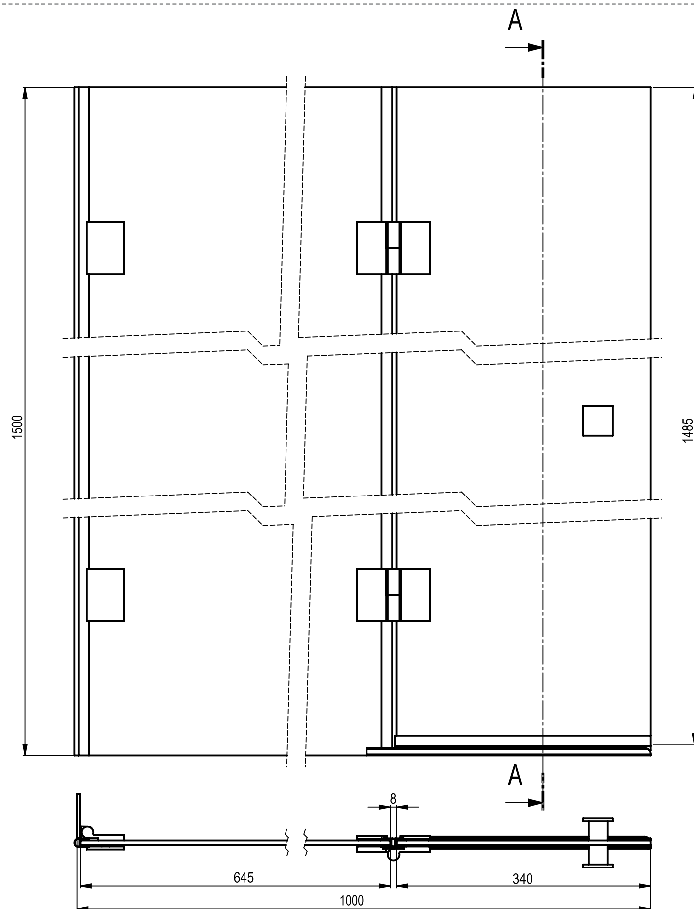
ŘEZ A-A
