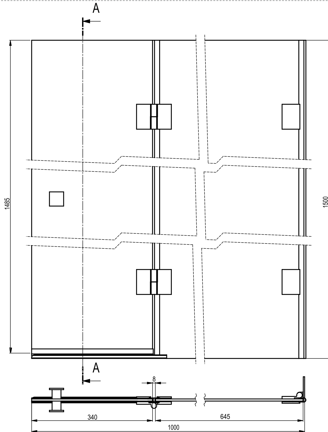
ŘEZ A-A
