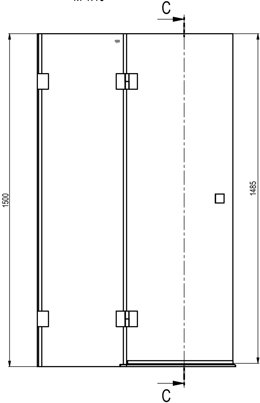
POHLED B M 1:10
