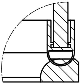
DETAIL D M 1:1
